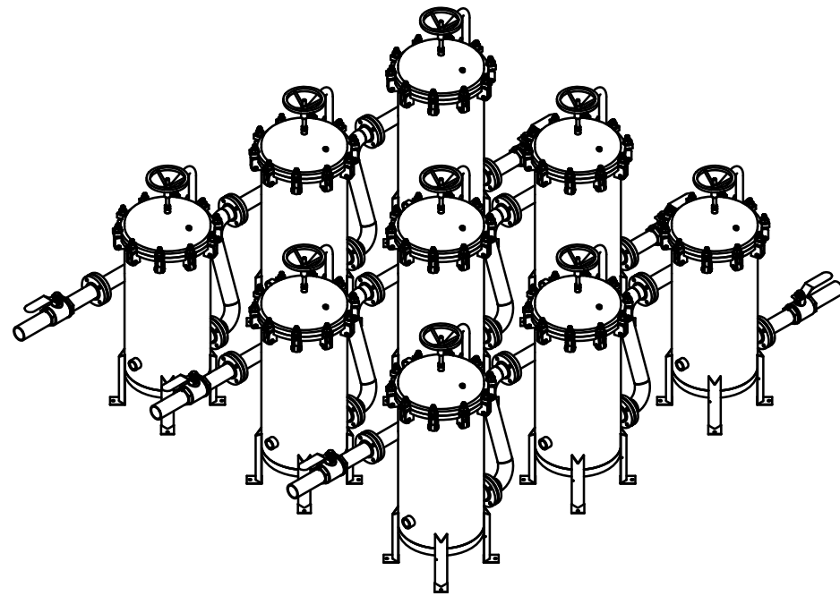
ИЗОМЕТРИЧЕСКИЙ ВИД
